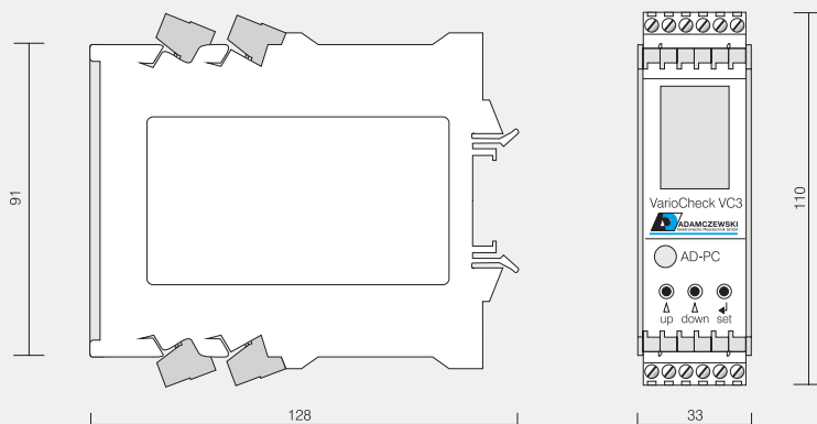
Abmessungen AD-VC 3 GVF
