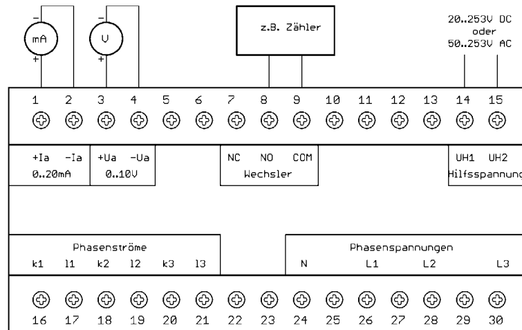
Abbildung 5: Anschluss Ausgänge und Versorgung
